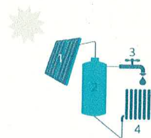
1 Zonnecollector | 2 Opslagvat zonneboiler | 3 Sanitair warm water | 4 Afgiftedrukt voor ruimteverwarming optimaal
